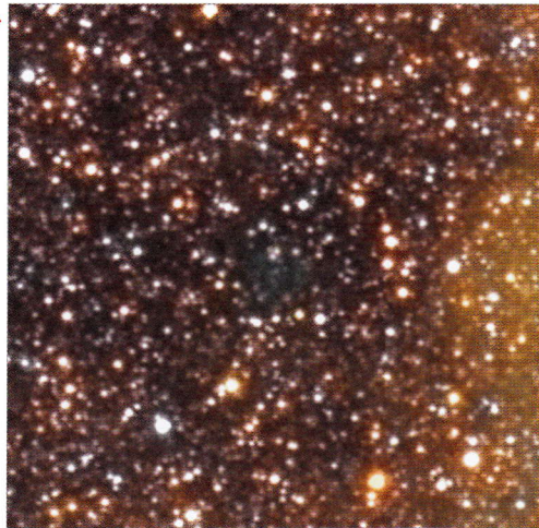
5. La nébuleuse planétaire probable DeGaPe 51.
