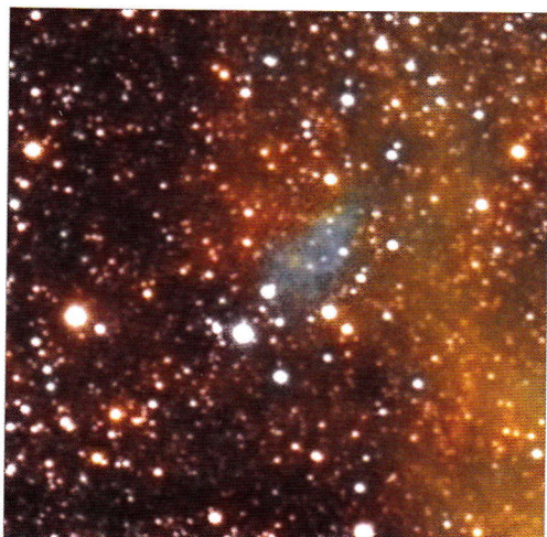
▲ 3. La nébuleuse planétaire probable DeGaPe 50.
