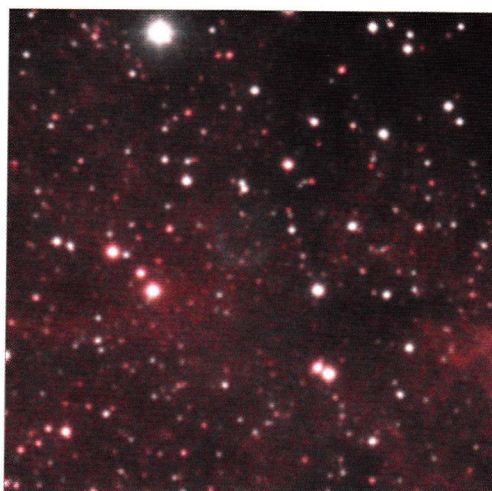
▲ 4. La nébuleuse planétaire probable DeGaPe 1.
